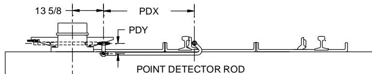
SECTION A-A POINT LUG
