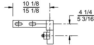
SECTION B-B SWIVEL LUG
